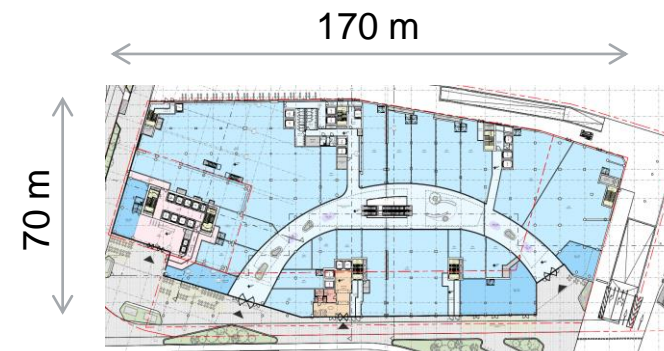
Tipični tloris Etaže 0–5
