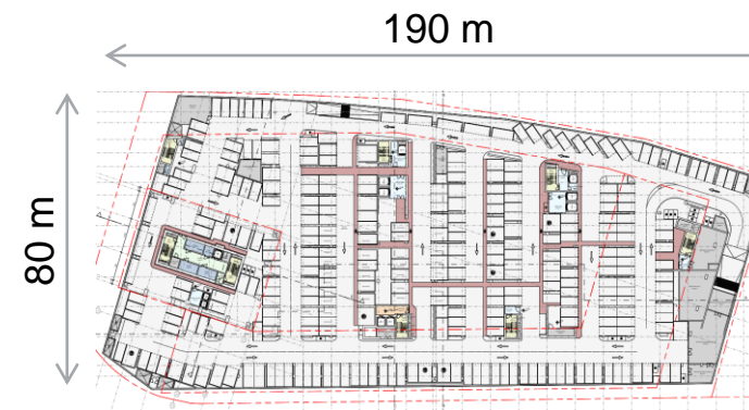
Tipični tloris Etaže -4 – -1
